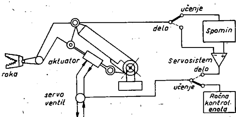
Slika 8: Industrijski robot
