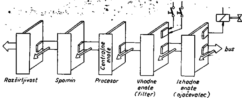
Slika 6a: Zasedba programirnega krmiljenja (PC)
