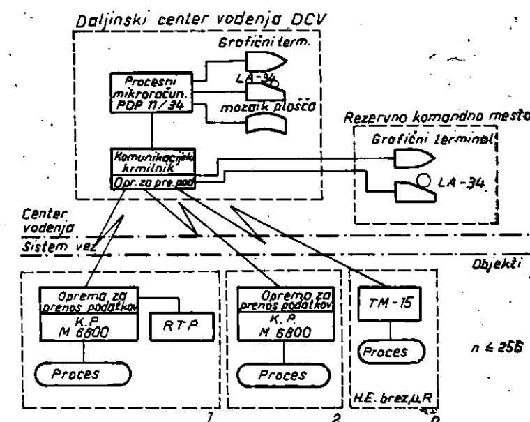
Slika 13: Hierarhična organizacija sistema za vodenje
