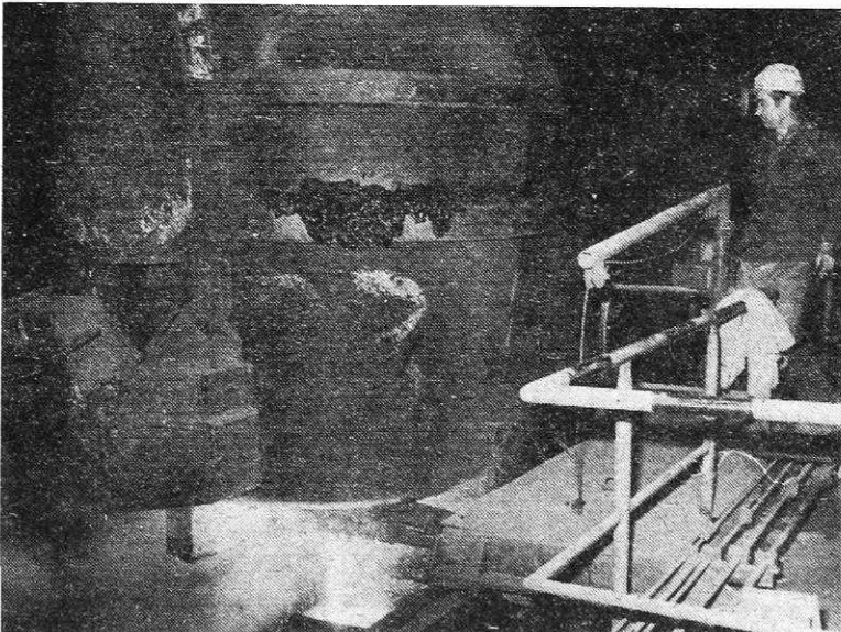
Vliivanje na konti-livu — Foto I. Kučina
