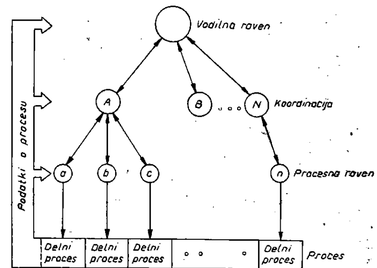
Slika 12: Osnovna struktura hierarhično organiziranega procesa
