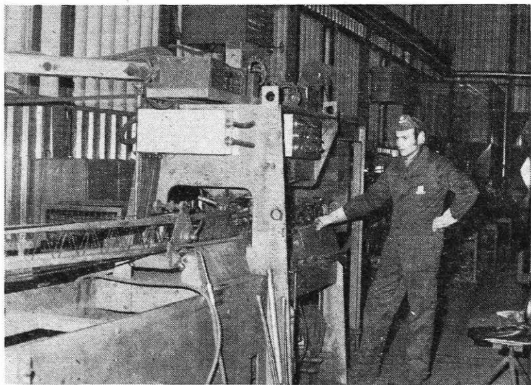
TOZD MONTER Dravograd – stroj za izdelavo statik nosilcev
