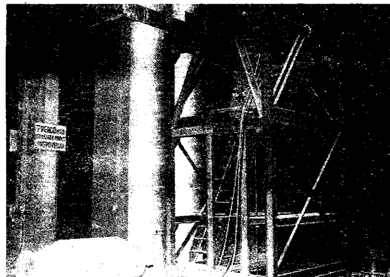
Novi naprava za vpihovanje CaSi praška na konti livu (Foto I. Kučina)
