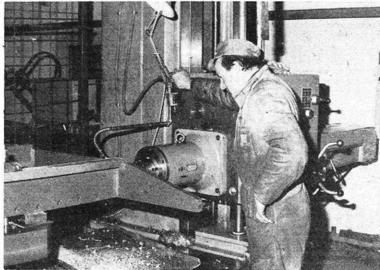
TOZD Monter Dravograd — horizontalni rezkalni stroj
