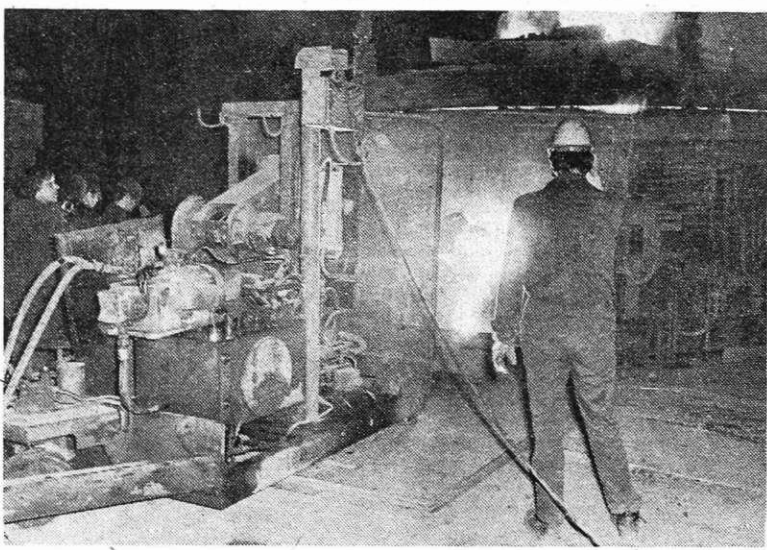
Vpihovanje kisika v SM peč (Foto S. Kokalj)
