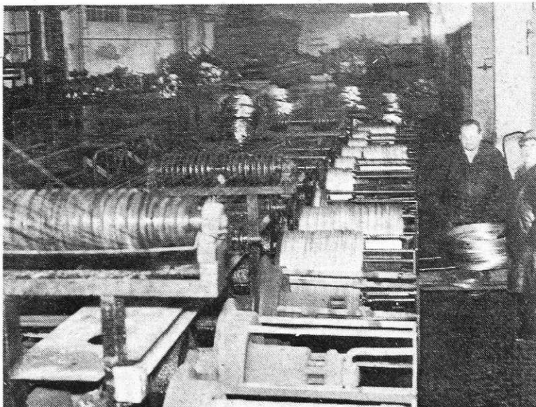
V lužilnici žice (Foto I. Kučina)
