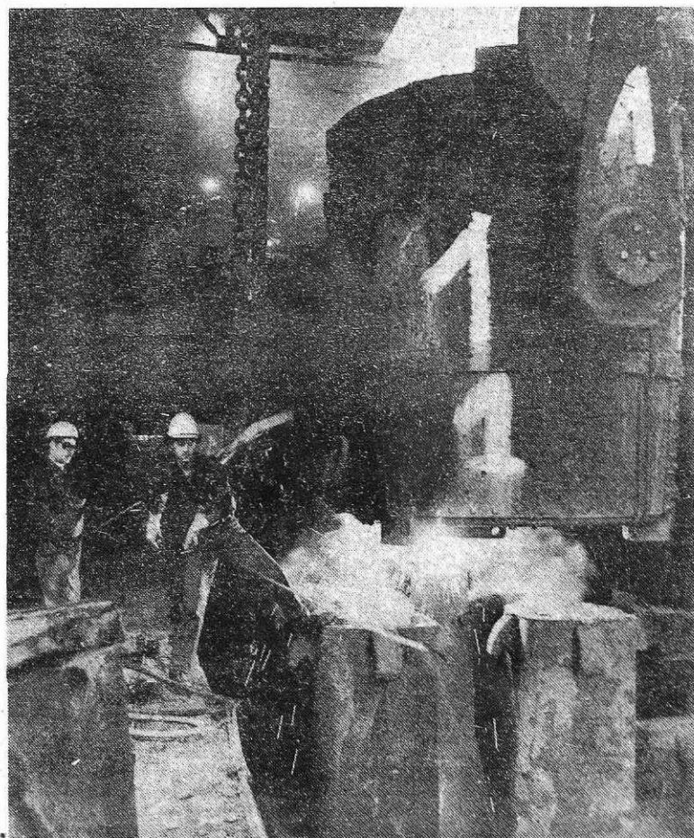
Vlivanje jekla (Foto I. Kučina)
