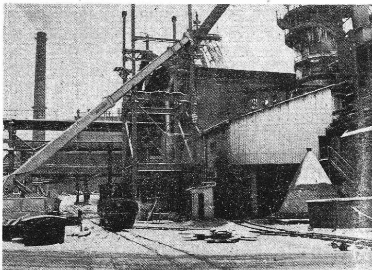
Montaža »prašne vreče« na plavžu (Foto I. Kučina)
