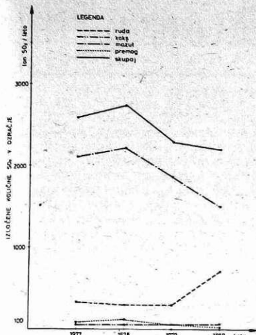
Diagram 1 — izločene količine žveplovega dioksida iz Železarne v ozračje jeseniške doline so iz leta v leto nižje
