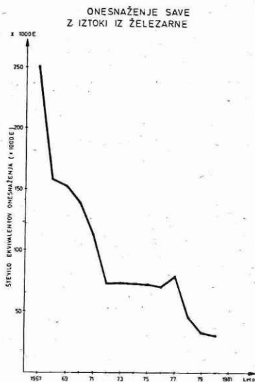
Diagram 3 — obremenitev Save z odplakami iz Železarne se je v zadnjih letih zelo zmanjšala, kar nam potrjujejo periodične analize onesnaženosti iztokov
