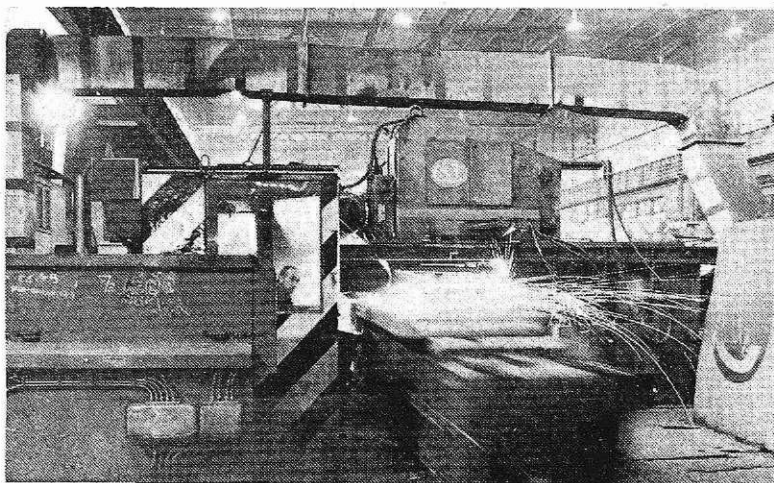
Površinska strojna obdelava jekla v valjarni bluming (Foto I. Kučina)
