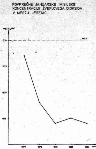
Diagram 2 — meritve, ki jih vsak dan izvaja Hidrometeorološki zavod SRS v centru Jesenic, kažejo, da so koncentracije žveplovega dioksida iz leta v leto nižje in celo v zimskem času le redko dosega dopustno mejo 0,3 mg SO 2 /kub. m.
