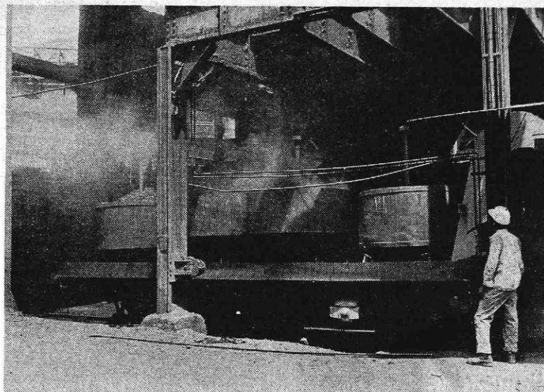
Polnjenje košar z rudo za zakladanje plavža (Foto I. Kučina)
