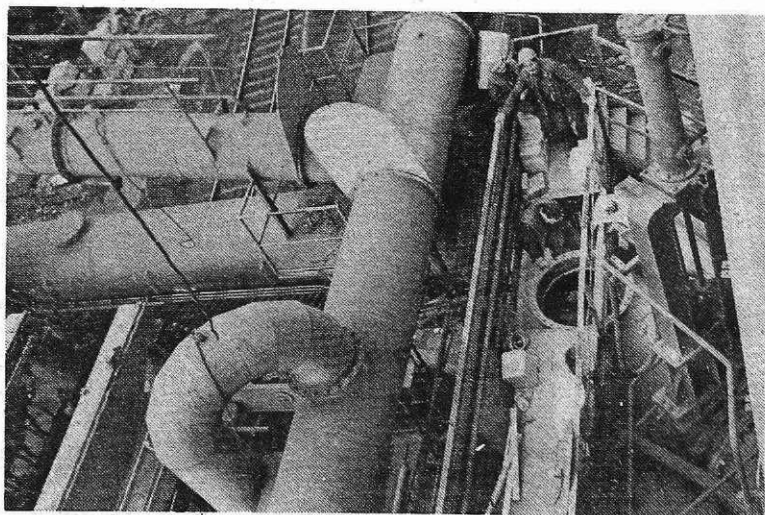
Obnova kaverperjev še vedno traja (Foto I. Kučina)
