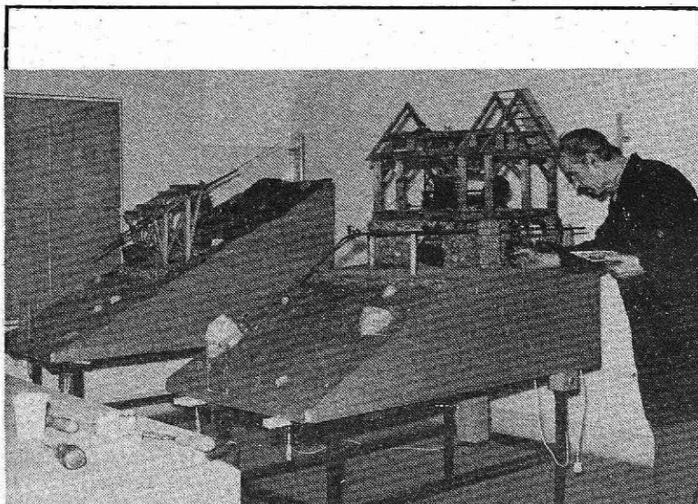
Nova pridobitev v tehničnem muzeju Železarne - Pantzova žičnica - izdelalek maketarja Marjana Dolinška (Foto I. Kučina)
