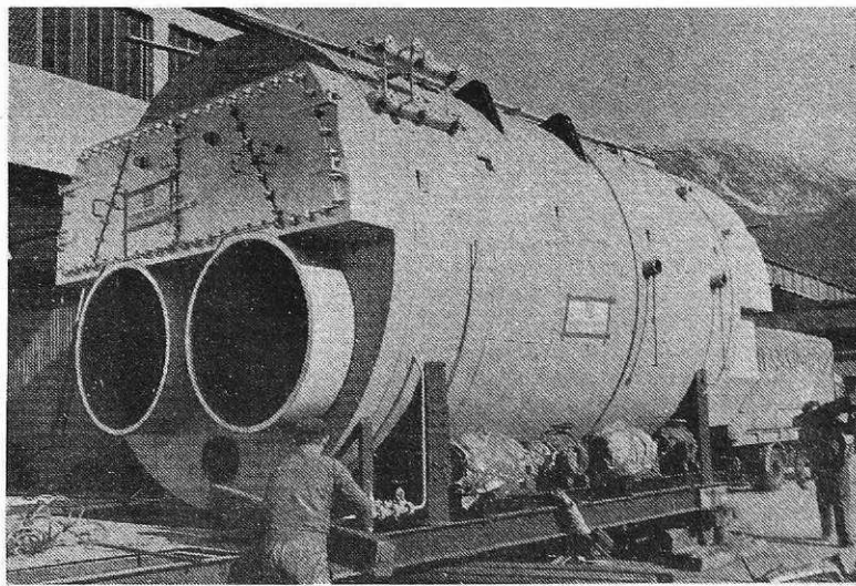
V roku je prispel parni kotel (25 ton/uro) iz podjetja Djuro Djaković za parno centralo na Beli (Foto I. Kučina)
