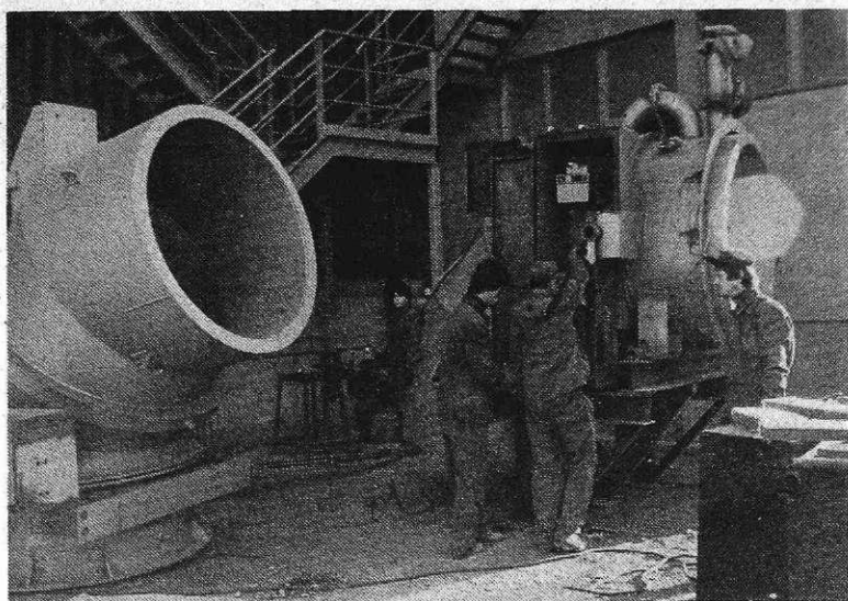
Montaža odpraševalnih naprav za odsesavanje četrte odprtine (Foto I. Kučina)
