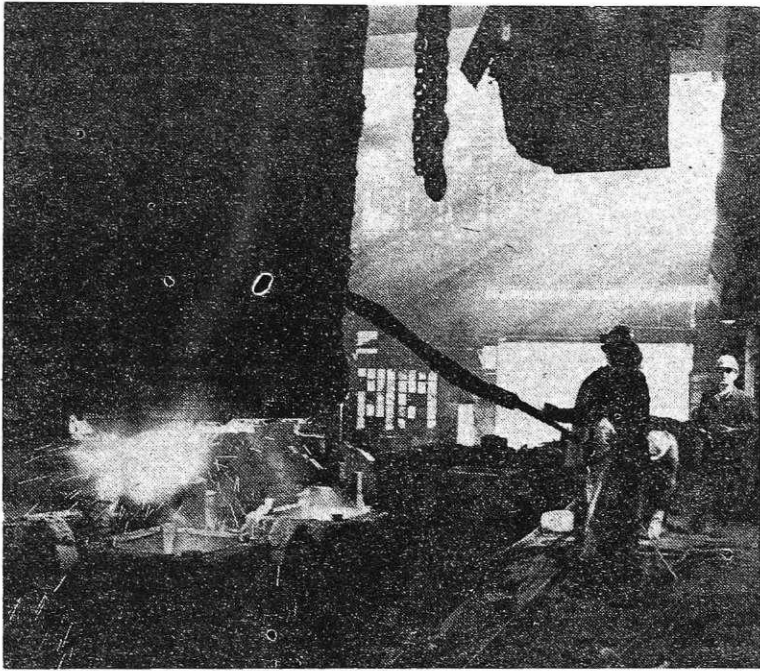
Kokile se polnijo z jeklom (Foto I. Kučina)
