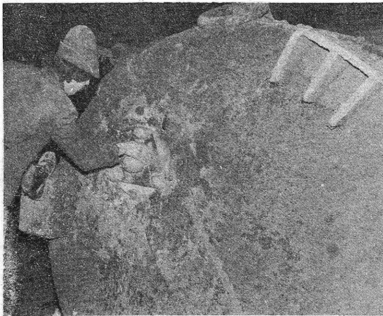
Obzidava dna ponve (Foto I. Kučina)
