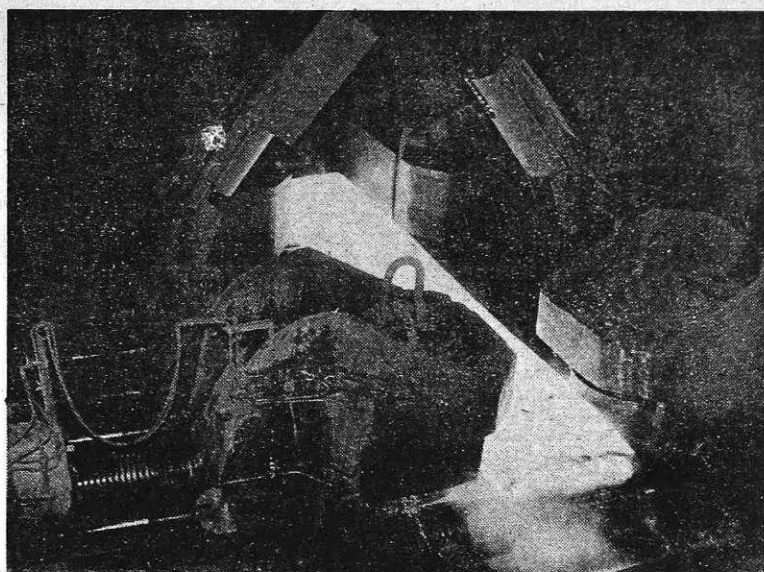
V valjarni bluming na Beli (Foto I. Kučina)
