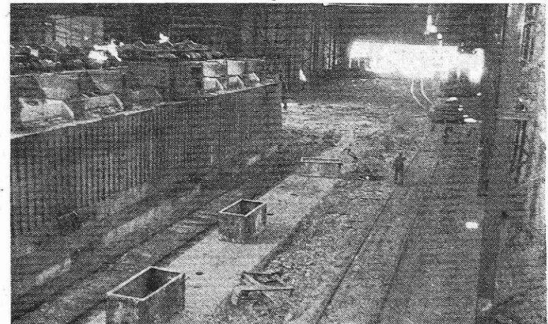
Hladnega vložka pred globinskimi pečmi v valjarni bluming-štel ni več (Foto S. Kokalj)
