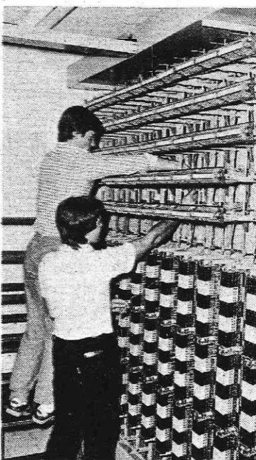
Vezava glavnega razdelilnika v novi avtomatski telefonski centrali (Foto S. Kokalj)
