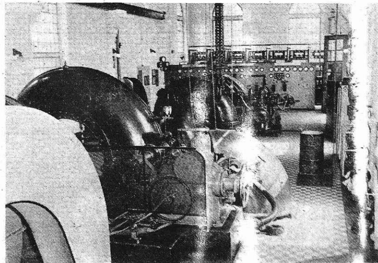
Notranjost hidroelektrarne v Zasipu (Foto S. Kokač)
