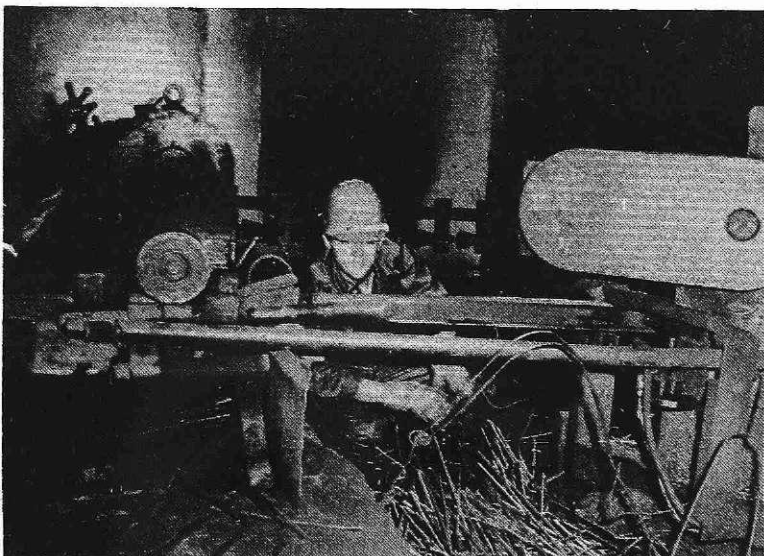
Sodelavec pri remontu valjarne žice (Foto S. Kokalj)
