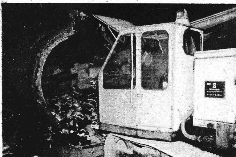
Strojno čiščenje ponvice (Foto S. Kokalj)
