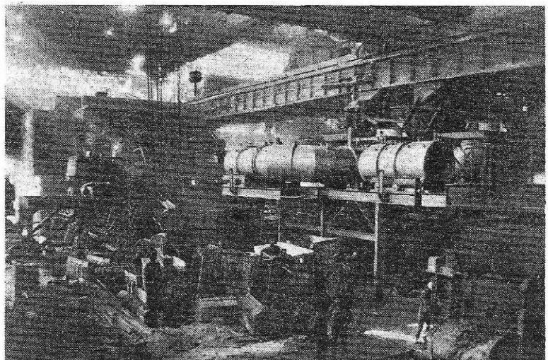
Remont ASEA električne peči in montaža odpraševalne naprave (Foto I. Kučina)
