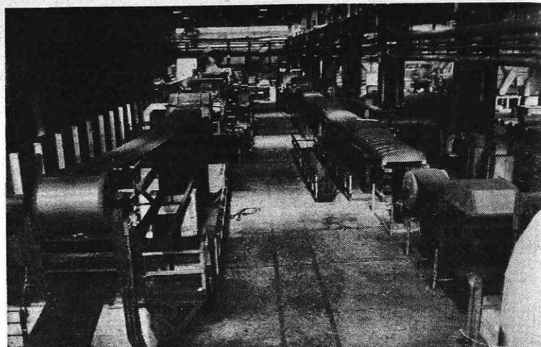
Žarilno-lužilna linija v Hladni valjarni Bela (Foto I. Kučina)
