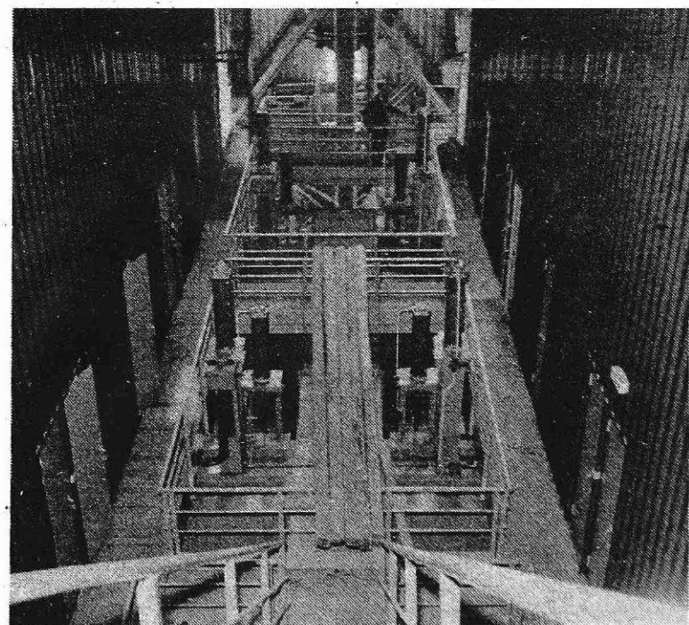
Novo odpraševalne naprave pri električnih pečeh (Foto I. Kučina)
