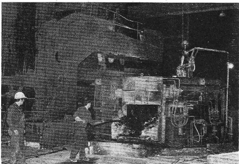
Zametovanje ASEA električne peči (Foto I. Kučina)
