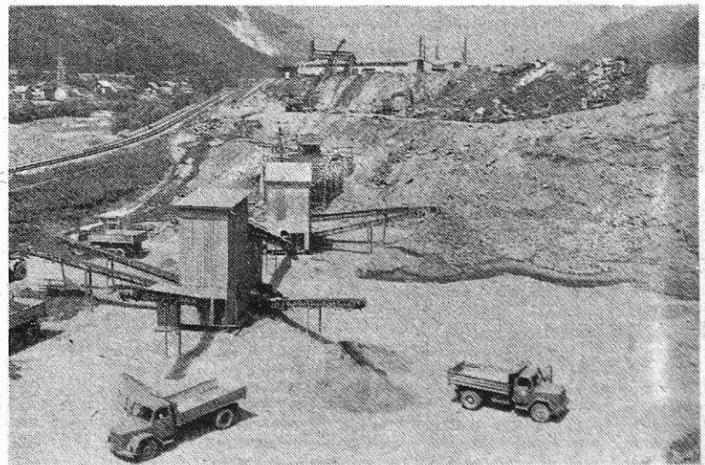
Separacija za žlindro
