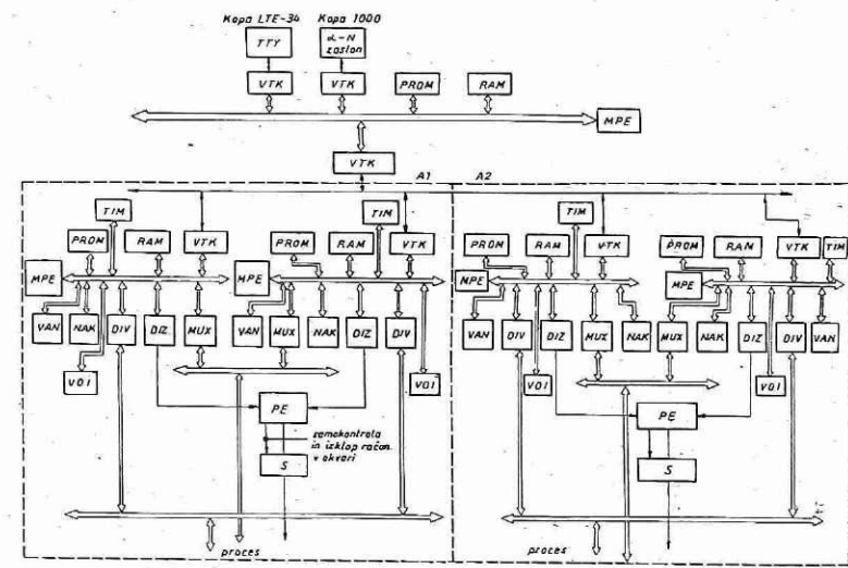
Slika 6: Moduli sistema za vodenje MHE
