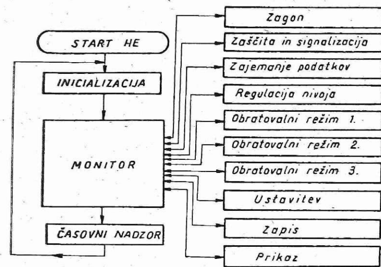
Slika 5: struktura programske opreme male hidroelektrarne
