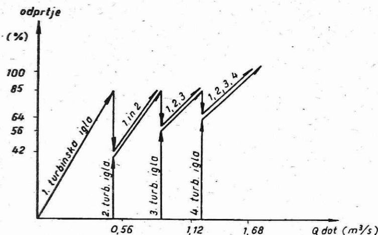
Slika 3: Zaporedno vklopljanje turbin
