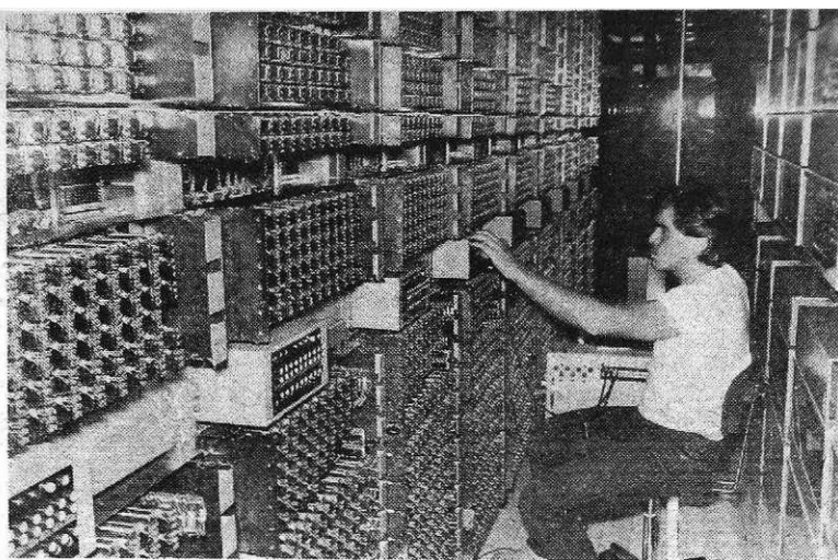
Testiranje nove telefonske centrale (Foto I. Kučina)
