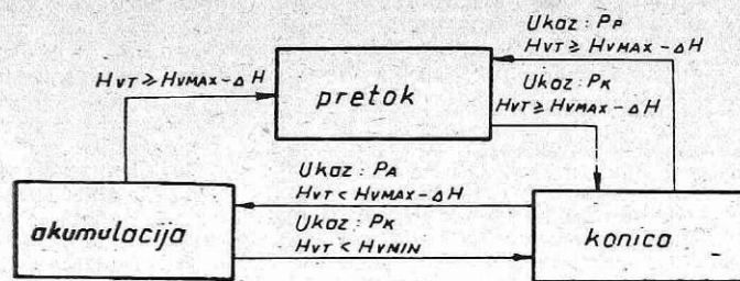
Slika 2: Obratovalna stanja in možni prehodi s stališča nivoja vode
