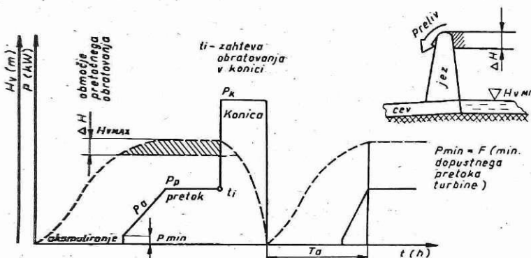
Slika 4: Dnevni diagram obratovanja male hidroelektrarne
