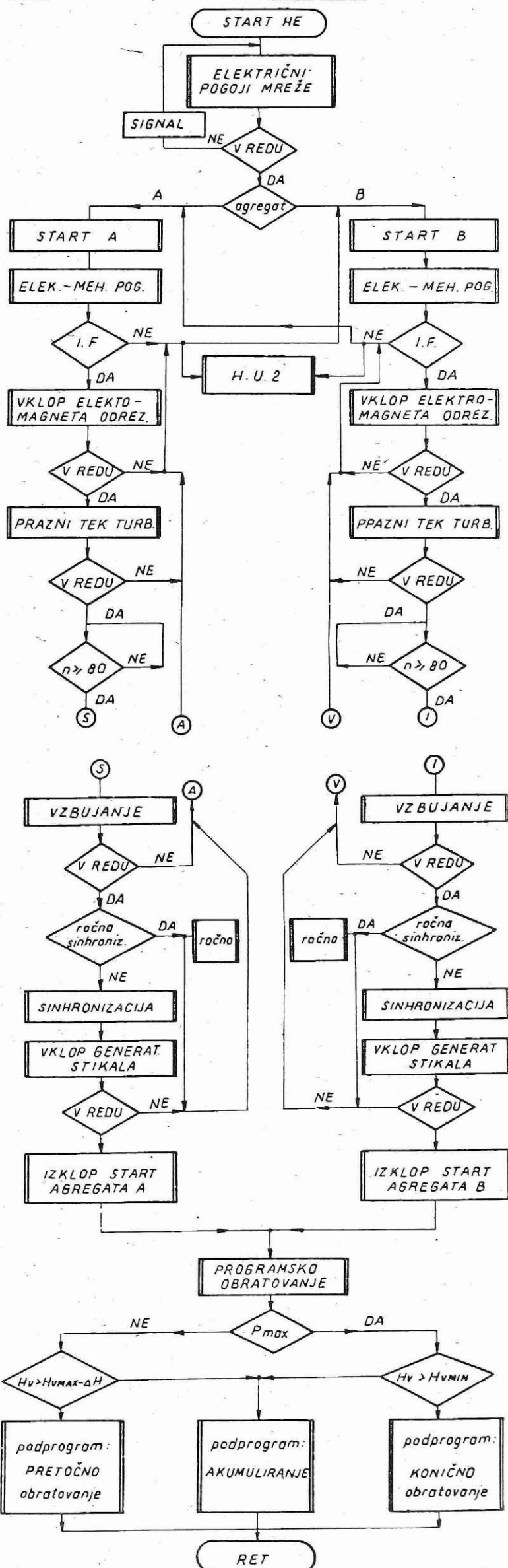
Slika 1: Diagram poteka zagona male hidroelektrarne
