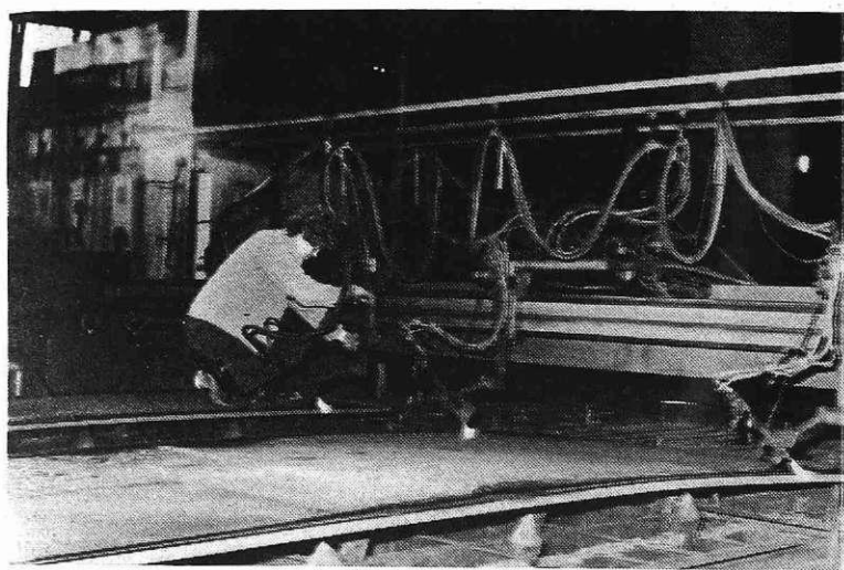
Autogeno rezanje debele pločevine (Foto I. Kučina)
