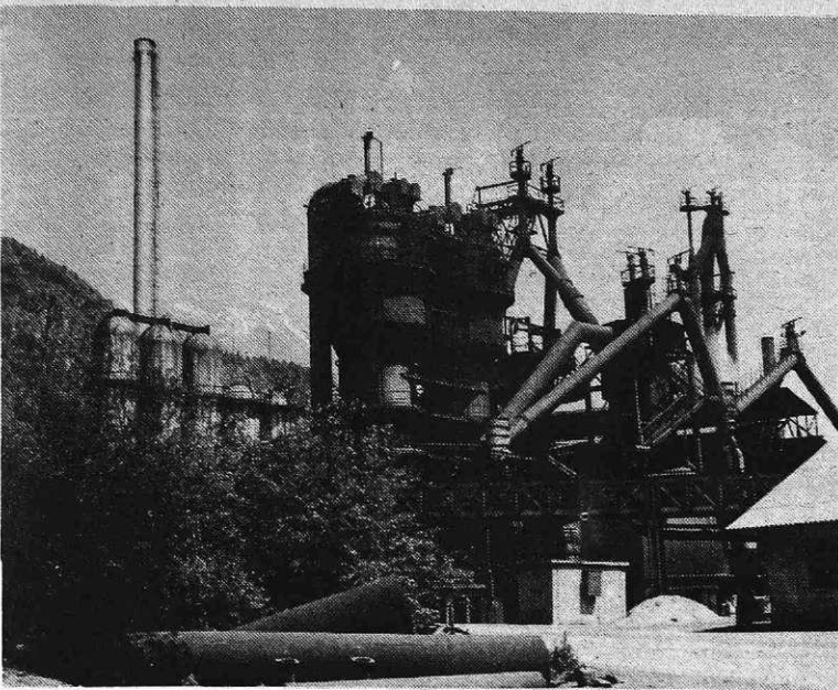
Plavža s kaverji (Foto I. Kučina)
