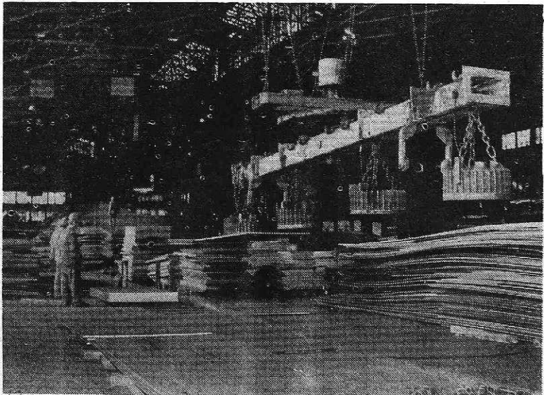
Adjustaža valjarne debele pločevine (Foto L. Kučina)
