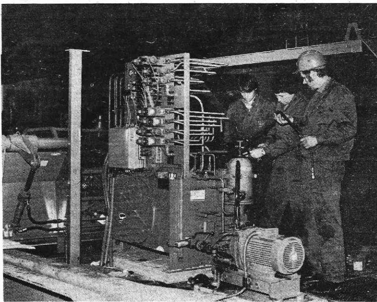
Montažna dela na novi profilni liniji v profilarni na Javorniku (Foto I. Kučina)
