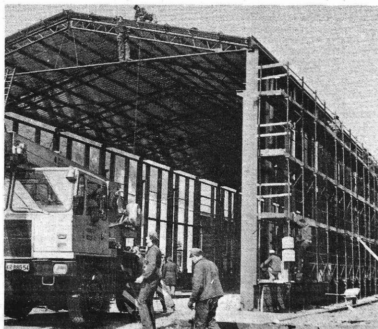
Pokrivanje in obzidava nove hale za elektrode (Foto I. Kučina)
