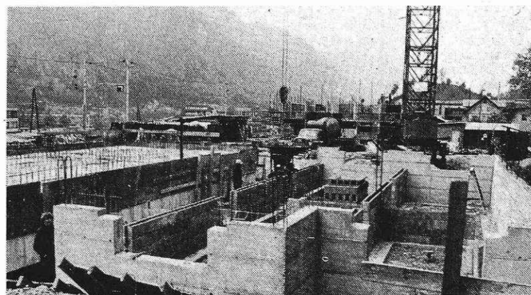
Gradnja stolpčev na Koroški Beli (Foto I. Kučina)
