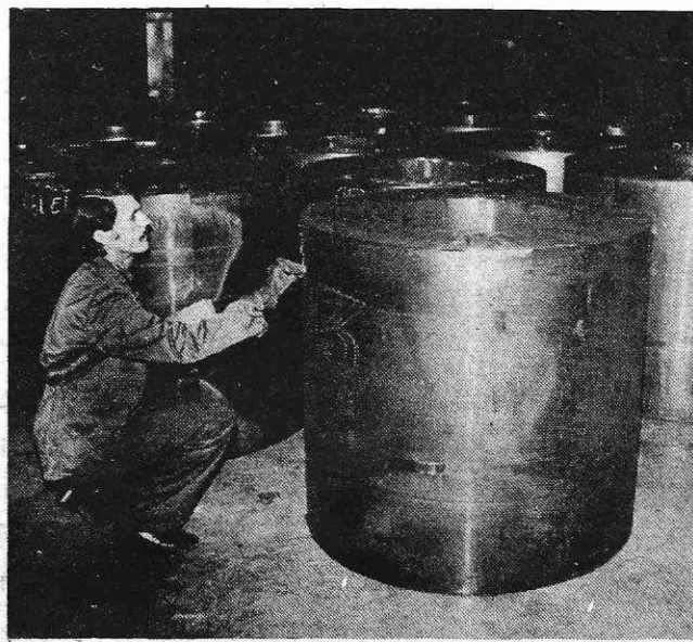
Signiranje pločevine v hladni valjarni Bela (Foto I. Kučina)
