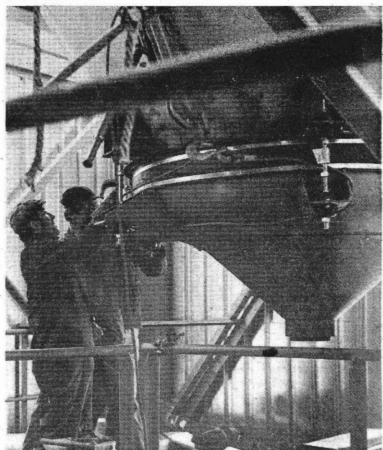
Montaža silosa za prah na novi odpraševalni napravi pri elektrojeklarni (Foto I. Kučina)
