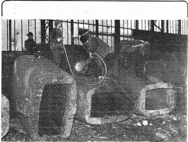
Priprava kokil v martinarni (Foto I. Kučina)
