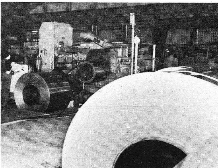
Previjalna linija v hladni valjarni Bela (Foto I. Kučina)
