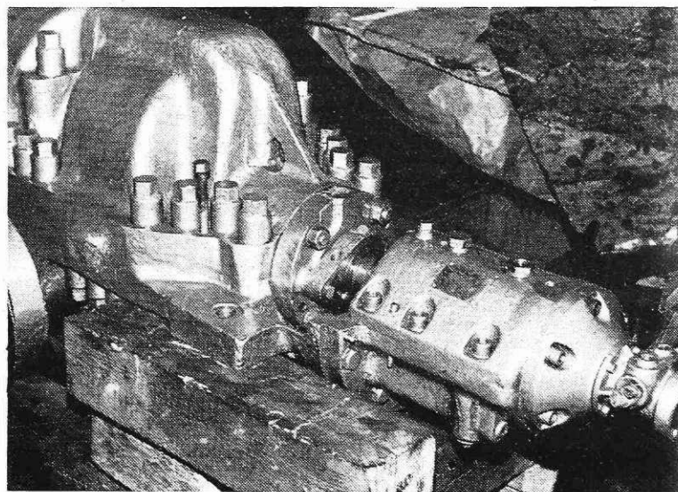
Popravljen ameriška črpalka z doma izdelanimi rezervnimi deli
