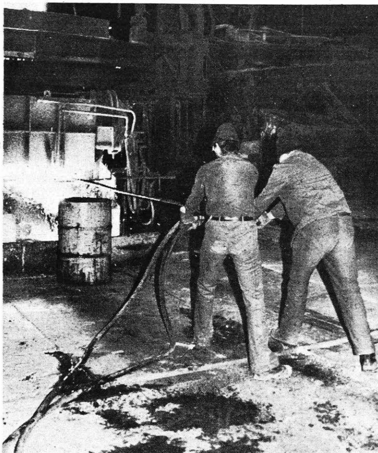
Sodelavca pri ASEA električni peči (foto I. Kučina)
