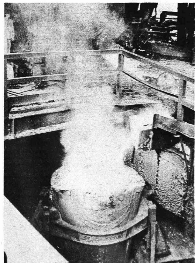
Izliv grodlja v ponvico (Foto I. Kučina)
