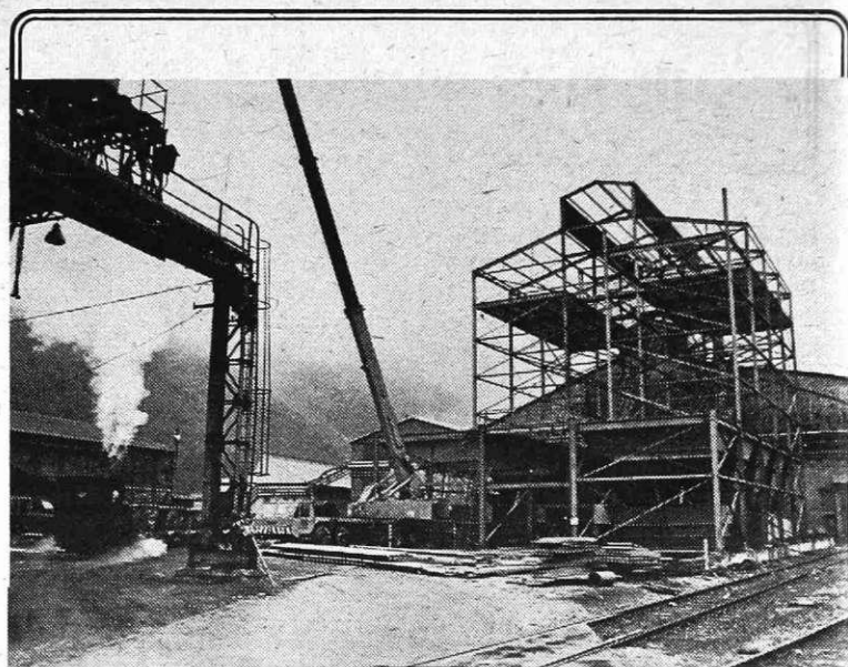
Gradnja novih odpraševalnih naprav (Foto I. Kučina)
