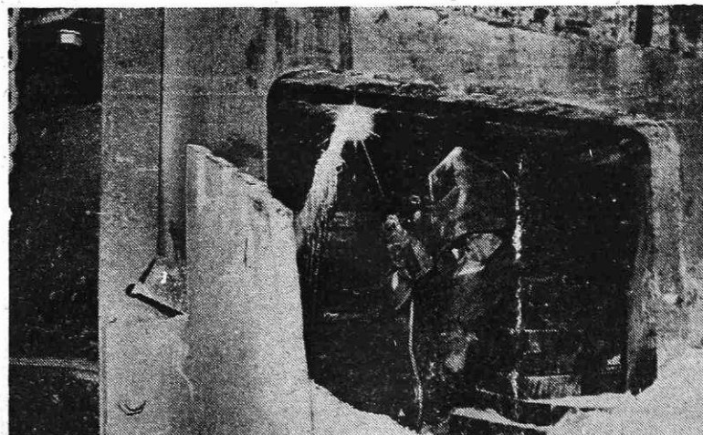
Remont na ASEA električni peči (Foto S. Kokalj)
