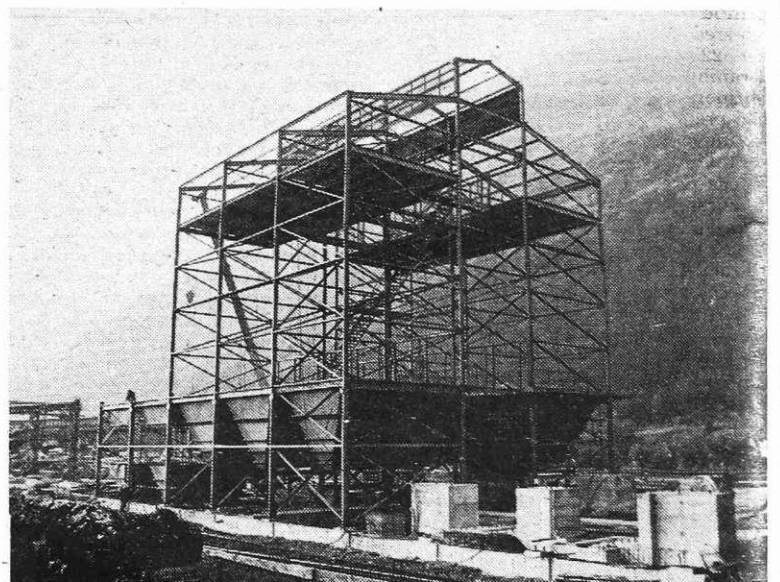
Del novih odpraševalnih naprav (Foto S. Kokalj)
