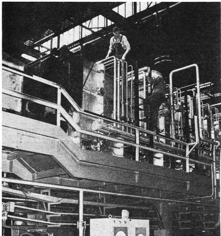
Priziganje žarilne peči v HVB (Foto I. Kučina)
