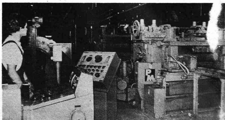
Linija za vzdolžni razrez hladno valjanih trakov (Foto I. Kučina)
