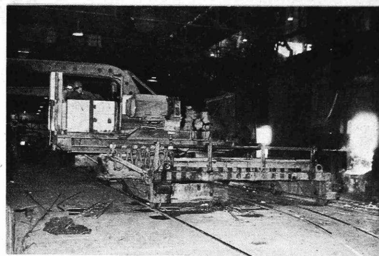
Zakladanje SM peči (Foto I. Kučina)
