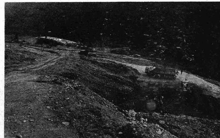
Gradbišče pred novim karavanjskim predorom na Belem polju (Foto I. Kučič na)
