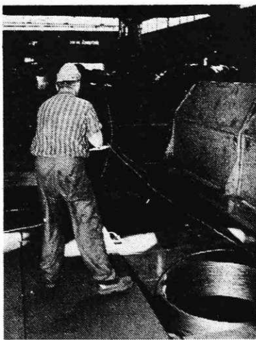
V valjarni žice (Foto S. Kokalj)
