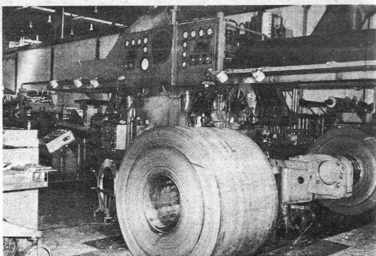
Previjalna linija v hladni valjarni Bela (Foto I. Kučina)
