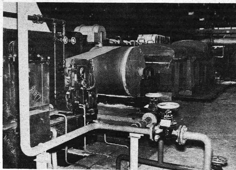
Lužilna linija v hladni valjarni na Beli
