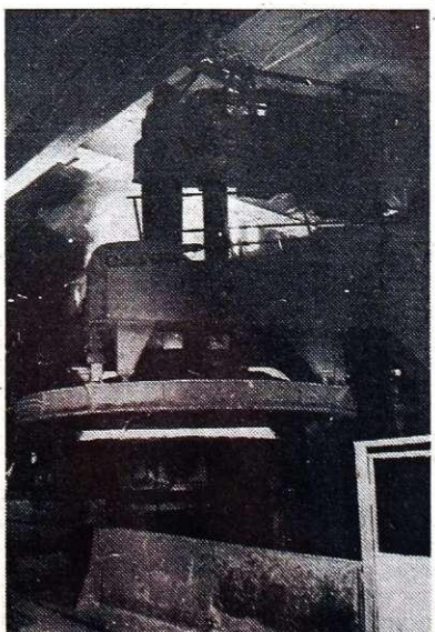
ASEA električna peč (Foto I. Kučina)
