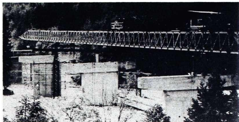
Delavci GIP Gradis uspešno napredujejo z graditvijo mostu čez Savo, kjer bo prišla na Belem polju nova cesta iz karavanškega predora. Kot vidimo tudi na sliki, je delo zelo zahtevno. Nosilni stebri so v glavnem postavljeni in tačas nanje stavljajo konstrukcijo, ki bo nosila štirinajst in pol metra široko cestišče. (Foto in tekst B. Blenkuš)
