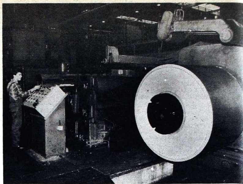
Žarilno lužilna linija v Hladni valjarni Bela (Foto I. Kučina)
