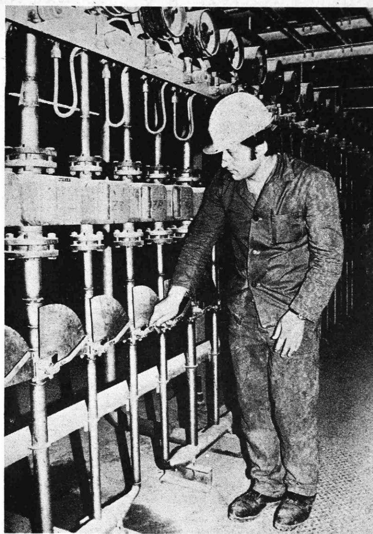
Sodelavec pri regulaciji izspiralne vode na konti livu (Foto I. Kučina)
