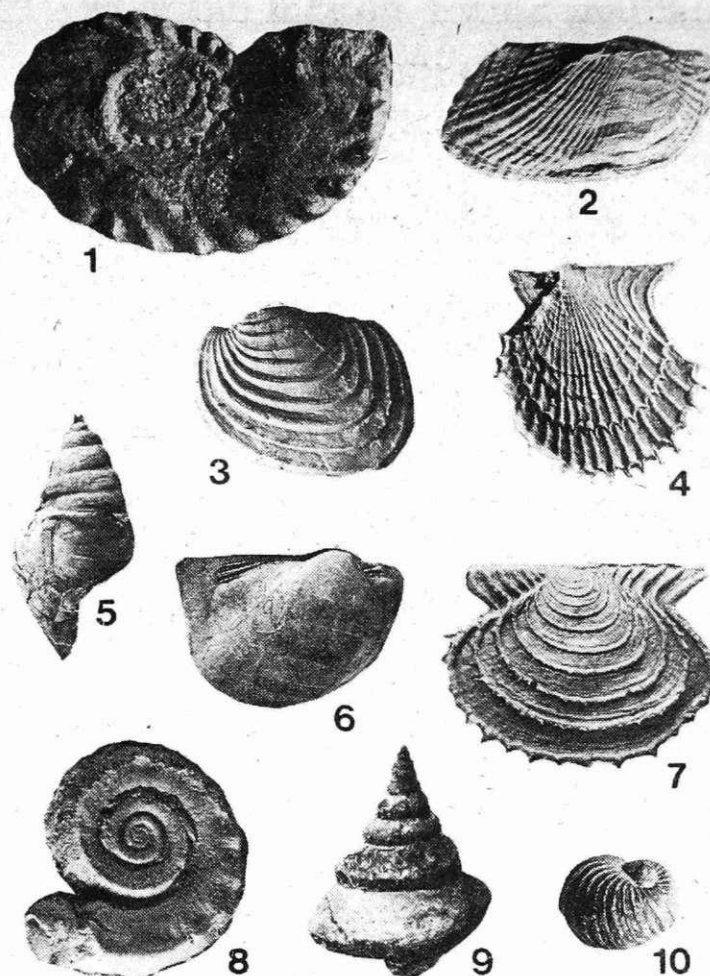
1. GLAVONOŽEC Gzheloceras sp. zg. karbon, Črni vrh, 2, 3, 4, 6, 7 ŠKOLJE: 2. Parallelodon javornikensis ; 3. Posidonia sp.; 4. Acanthopecten carboniferous ; 6. Cucullopsis quadrata jugoslavica; 7. Annuliconcha spinosa . Vse zgornji karbon, Javorniški rov; 5, 8, 9, 10 POLŽI: 5. kamnito jedro zgornjekarbonskega polža, Javorniški rov; 8. Euomphalus sp., spodnji permij, Pristava; 9. Omphalotrochus sp., spodnji permij, Na pečeh; 10. Natiria costata , spodnji trias, Spica v Sedelcih. (Sl. A) — (Foto Jože Bedič)
