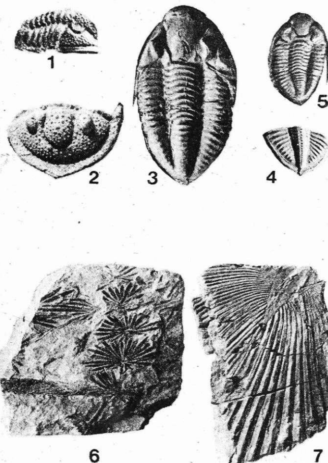
1. — 5. TROKRPARJI 1. in 2. Brachymetopus pseudometopina . Cel primerak od strani in glava; 3. Paladin (Kaskia) bedici; 4. Pseudophilipsia (Carniphilipsia) rakoveci, zadek. Vse zgornji karbon, Javorniški rov; 6. Annularia stellata , zgornji karbon, Golica; 7. Palma iz rodu Sabal sp. eocen, Lepene. (Sl. B) — (Foto Jože Bedič)
