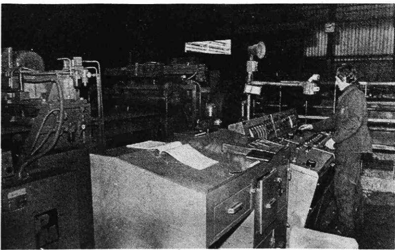
Izstopni del lučilno-žarilne linije v HVB (Foto I. Kučina)
