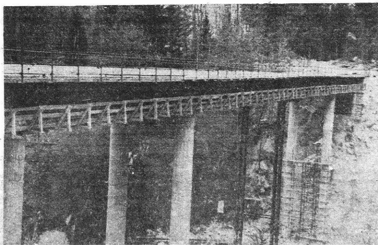
Nov most čez Savo Bohinjsko na Ohrnah (Foto: B. Blenkuš)
