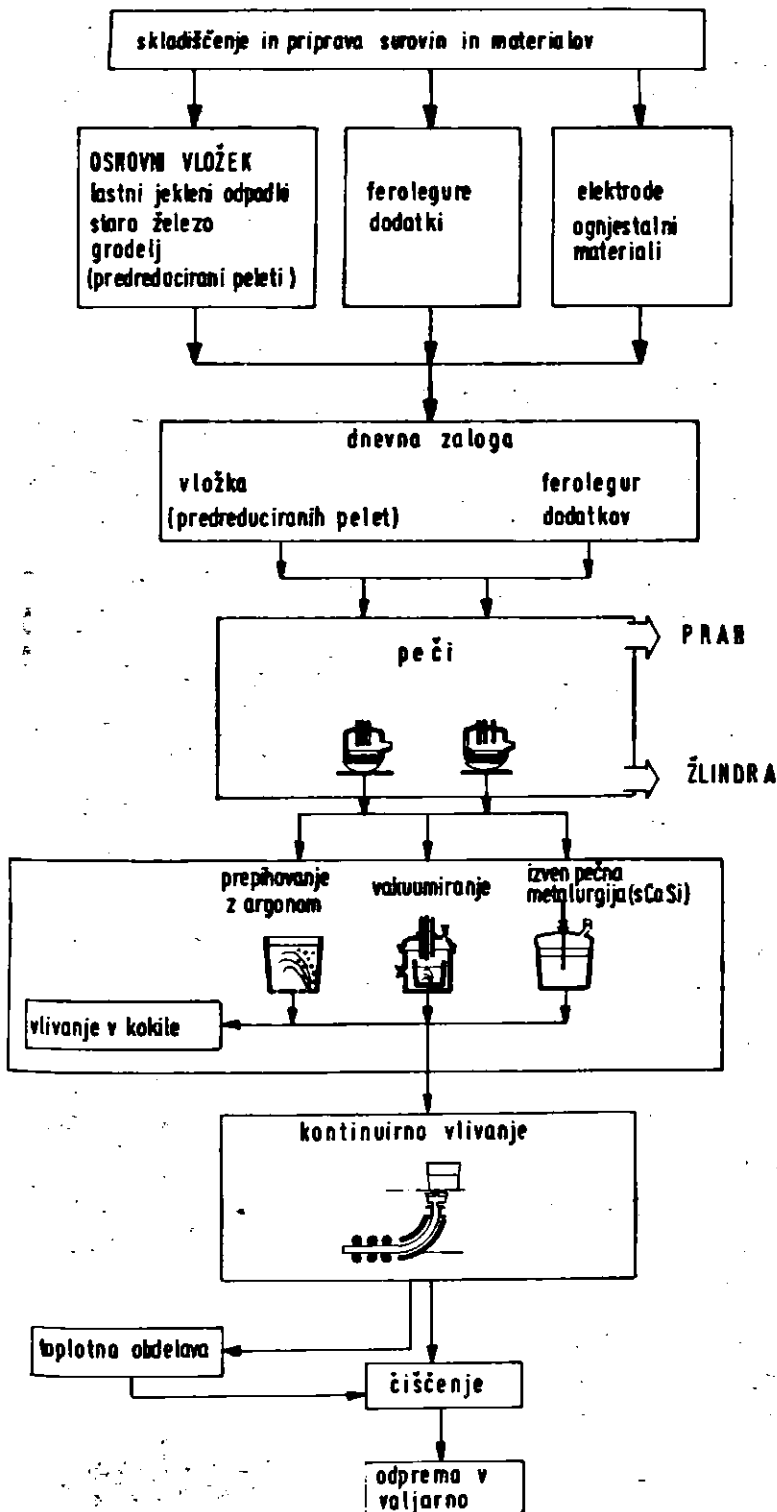
Slika 1 SHEMA TEHNOLOŠKEGA POSTOPKA
