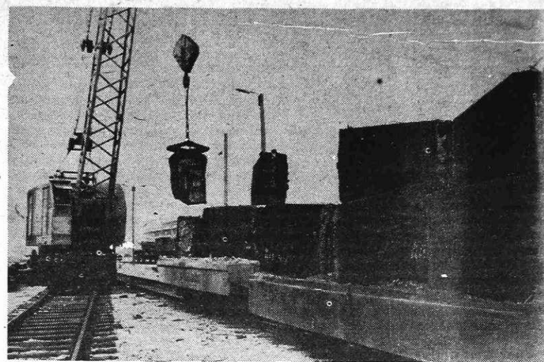
Vložek za valjarno bluming (IK)
