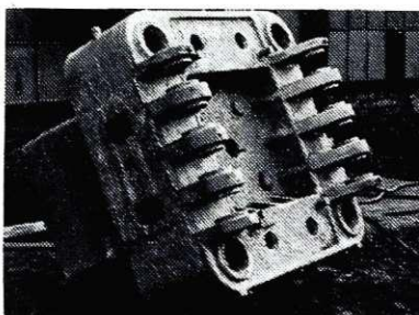
Ulitek za stiskalnice GDK 900 Weingarten
