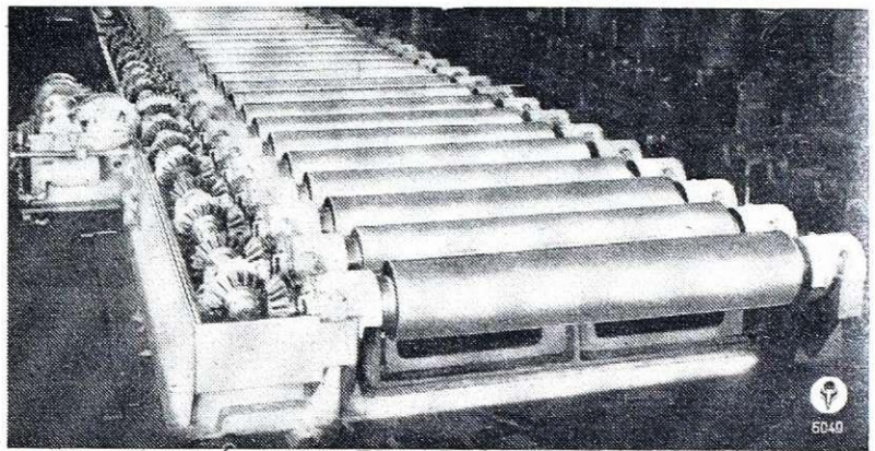
500 ton ulitkov vseh vrst je bilo napravljeno v naši livarni za Valjarno bluming na Beli
