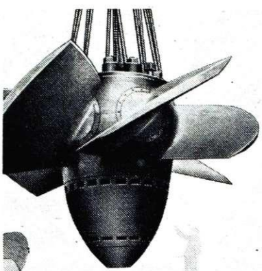
Naš ulitek — glava kaplanove turbine vgrajen v tekač turbine v Srednji dravi I. teža 45 ton, celotni tekač tehta 350 ton
