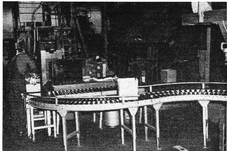
Pakiranje žičnikov v žebliarni (SK)
