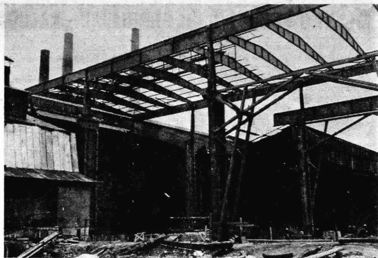
Gradnja hale za konti-lij
