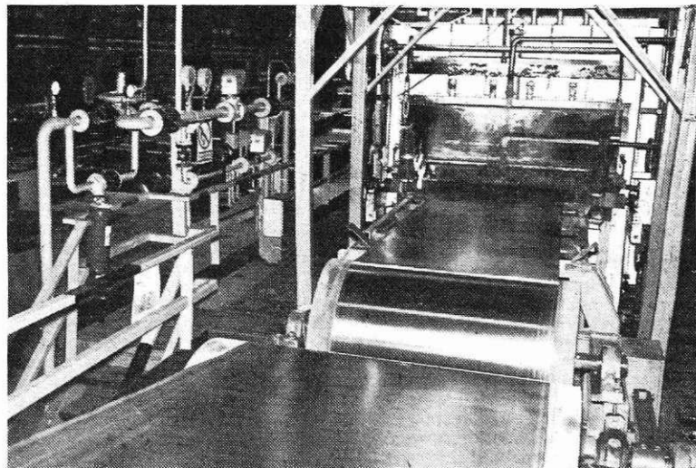
Del žarilne linije v HVB
