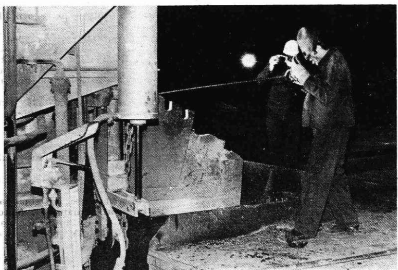
Sodelavci pri ASEA električni obločni peči
