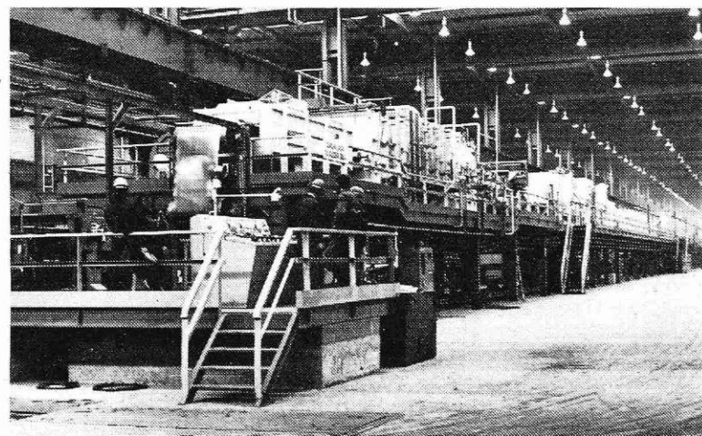
Žarilna linija za silicijeva jekla v HVB
