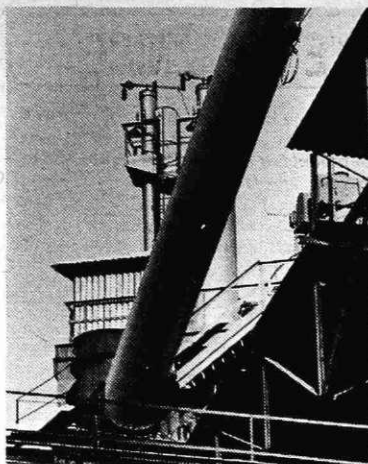
Montaža novega plinovoda za plavž
