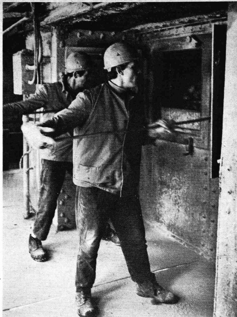
Sodelavca na apnenici pri peči za izdelavo žganega apna
