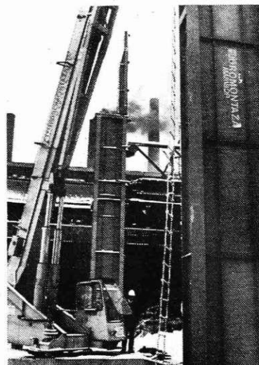
Postavljanje drugega nosilnega stebra za konti-liv
