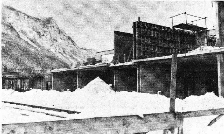
Gradnja šolskega centra na Plavžu
