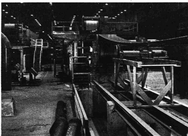
Žarilno-lužilna linija v hladni valjarni Bela
