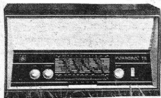
Slika 3: Kako pogosto poslušate radio?
