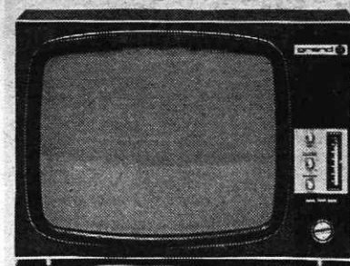
Slika 4: Kako pogosto gledate televizijo?
