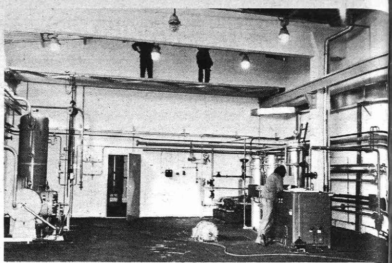
Strojnica vodikarne — valjarne Bela
