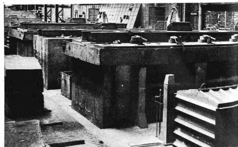
Zvonaste žarilne peči v valjarnah Javornik za sferoidizacijsko žarenje jekel za kvalitetne vijake
