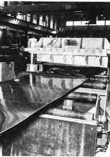
Škarje za vzdolžni prerez pločevine za nerjavna in ogljikova jekla
