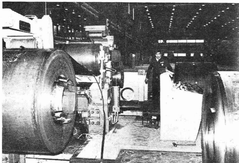
Previjalna linija v hladni valjarni Bela
