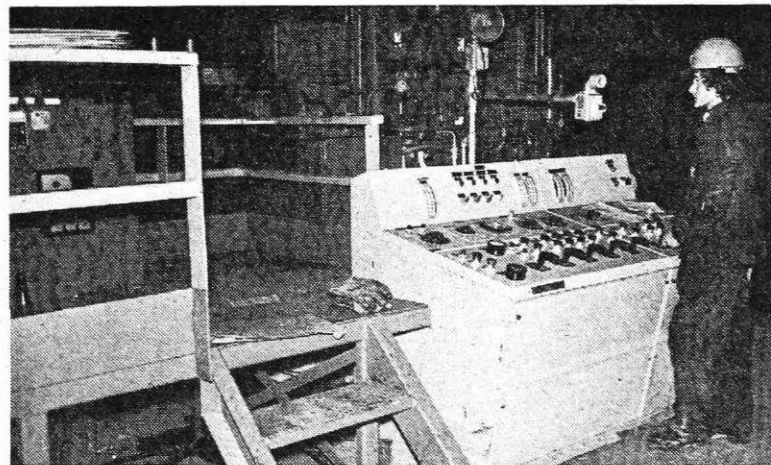
Vstopni del v žarilno lužilni liniji hladne valjarne Bela
