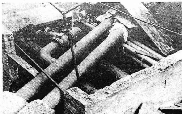
Prejšnji teden so delavci IMP Ljubljana v sodelovanju z delavci toplotne energije Železarne pri gimnaziji priključili nov toplovod na že obstoječe omrežje in preizkusili delovanje istega.
