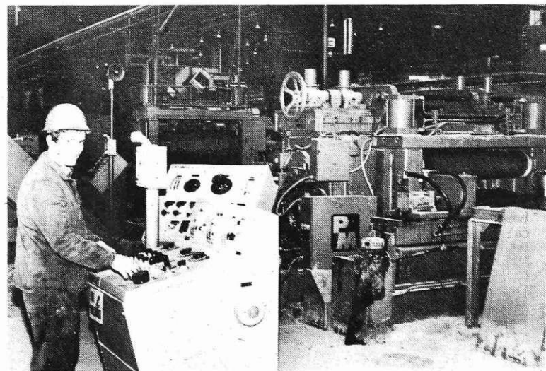
Linija za pripravo trakov z glavnim komandnim pultom v hladni valjar- ni Bela
