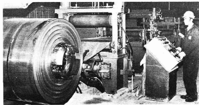
Testiranje vzdolžnih škarij s pločevino za nerjavna in ogljikova jekla
