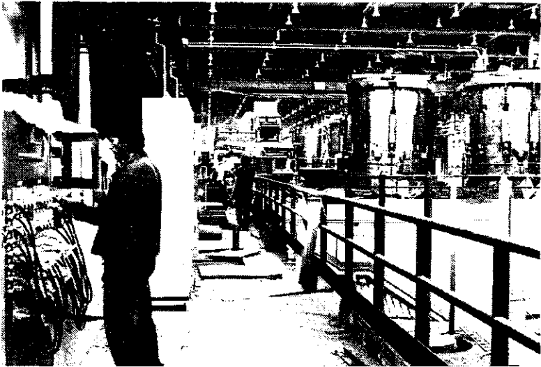
Aparatura za žarilne peli v novi hladni valjarni
