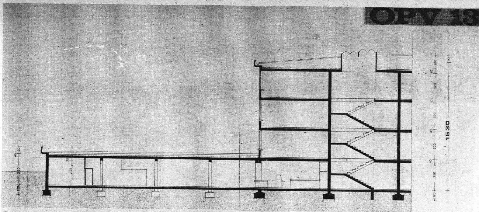
PREREZ B-B
