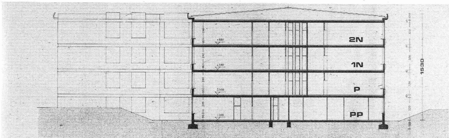
PREREZ A-A
